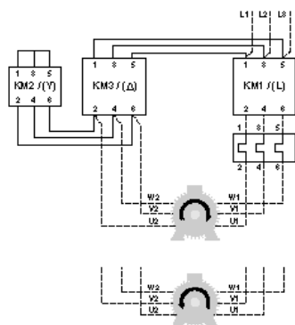
Схема силовой цепи
